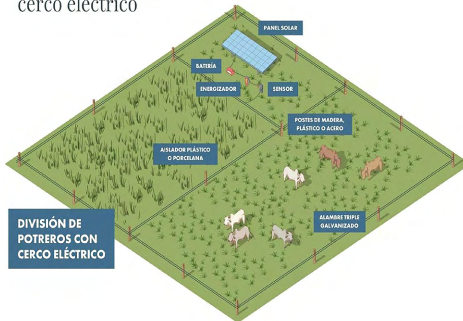
Figura 6. Componentes de los cercos eléctricos. Fuente: CONSELVA Costas y Comunidades, A.C.
